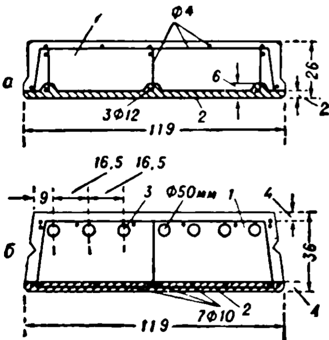
Рис. 3. Поперечные разрезы плит из ячеистых бетонов для чердачных (а) и бесчердачных (б) покрытий жилых зданий: 1 — ячеистый бетон; 2 — обычный бетон; 3 — вентилярующие продухи (осушающие каналы) диаметром 50 мм.
