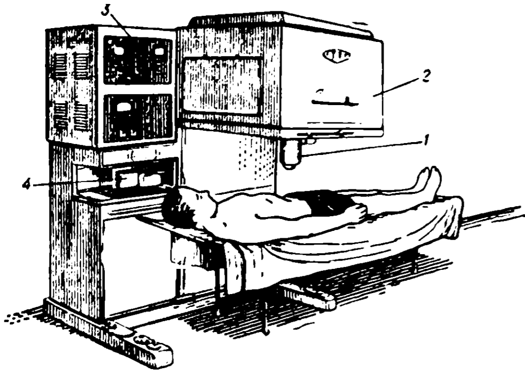
Рис. 1. Гамматопограф GT-60: 1—сцинтилляционный счетчик в защитном свинцовом кожухе; 2—механизм сканирования (под кожухом); 3—электронный блок; 4—регистрирующее устройство.
