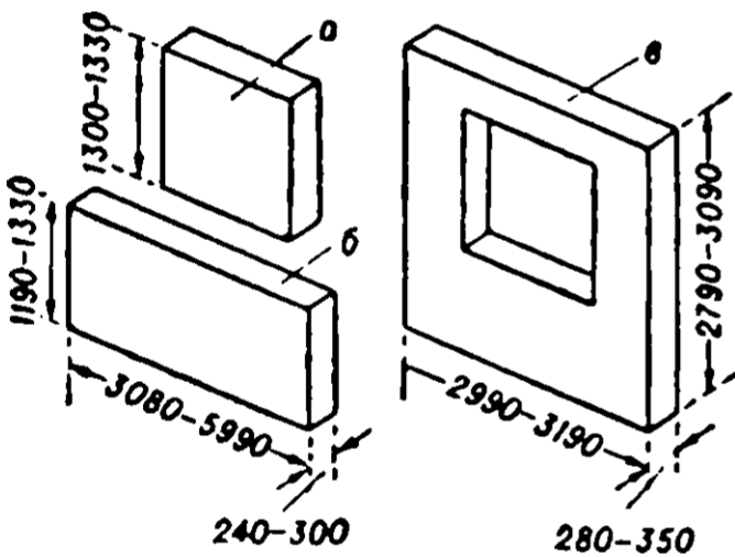
Рис. 2. Крупноразмерные элементы из ячеистого бетона для жилых зданий: а — простеночный; б — поясной; в — панель «на комнату».
