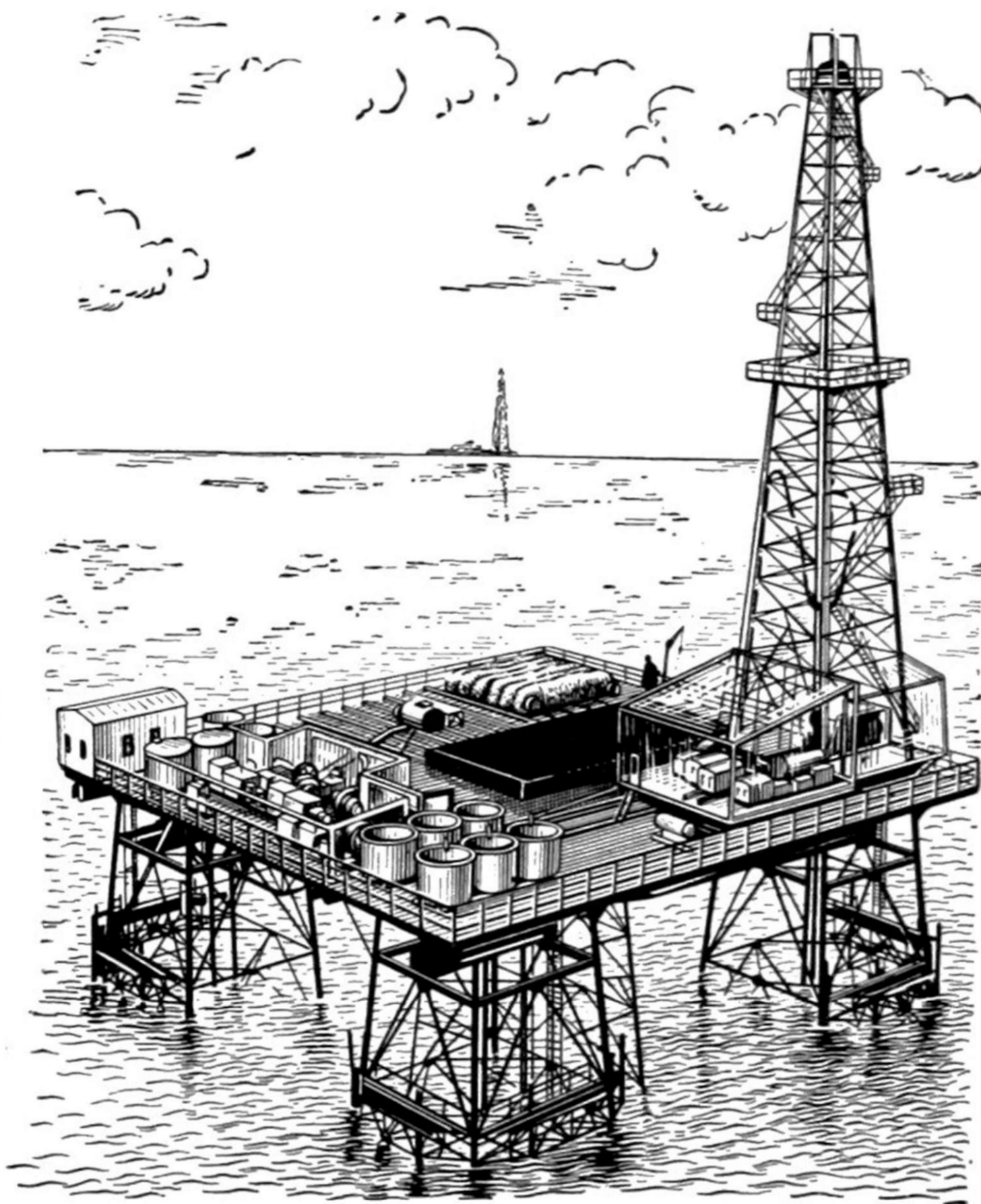
Глубоководное морское основание для разведки и разработки нефтяных месторождений при глубине моря 60 и более метров.
