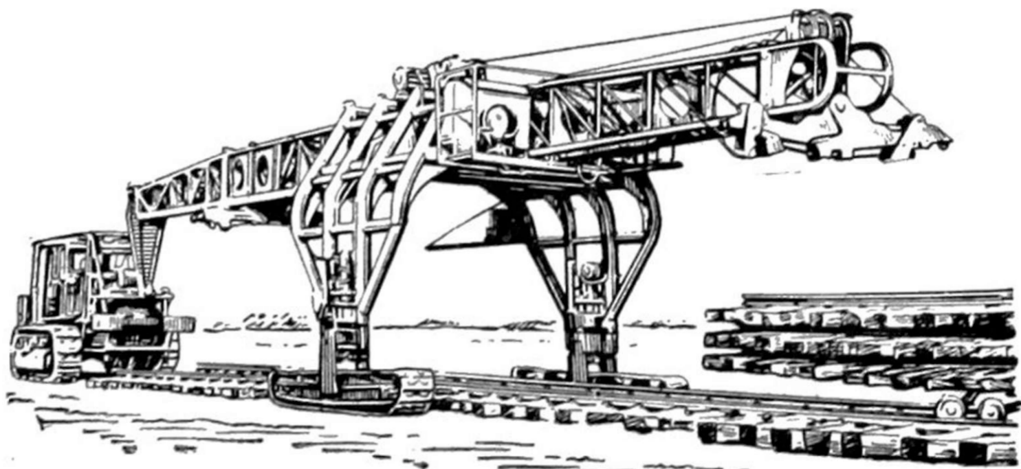
Рис. 3. Укладка пути звеньями длиной 25 м тракторным порталным путьукладчиком.
