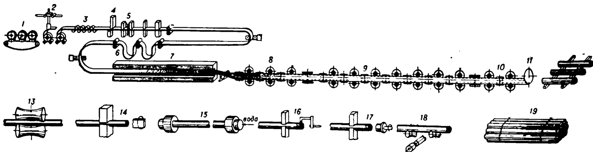
Принципиальная схема стана непрерывной печной сварки труб.
