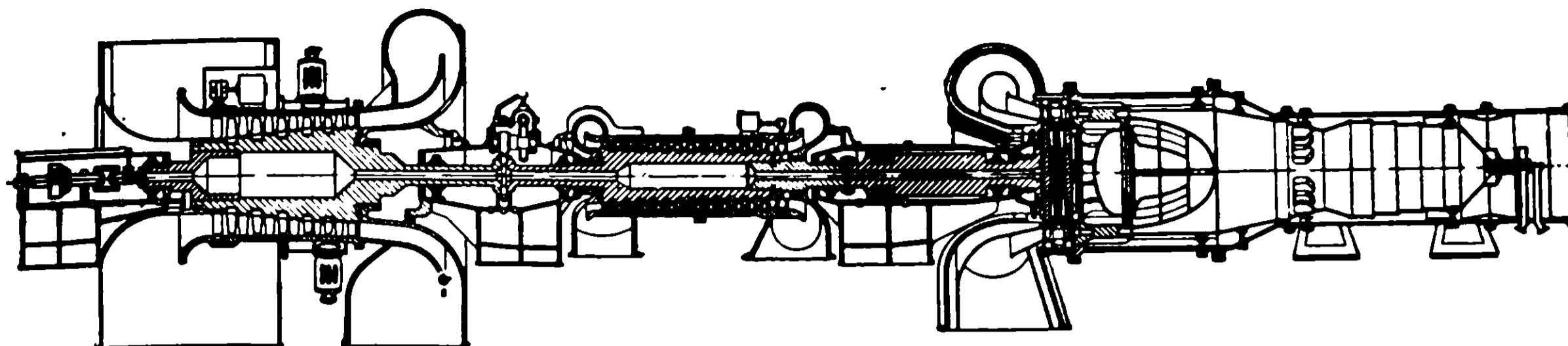
Рис. 1. Газотурбинный агрегат 50 000 квт. Продольный разрез компрессора низкого давления, компрессора высокого давления, турбины высокого давления и камеры сгорания высокого давления.
