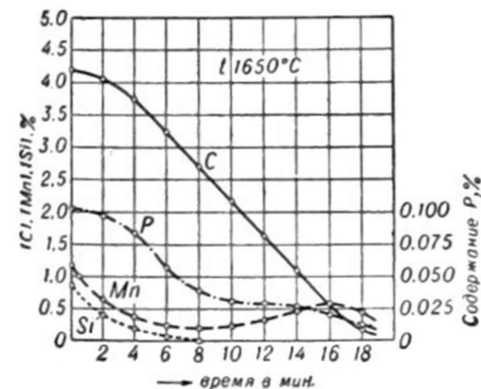
Рис. 2. Изменение состава металла при продувке в конвертере.
