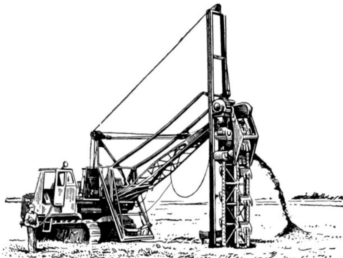
Рис. 1. Рытье котлованов под опоры контактной сети МКТС-2 на тракторе С-100.
