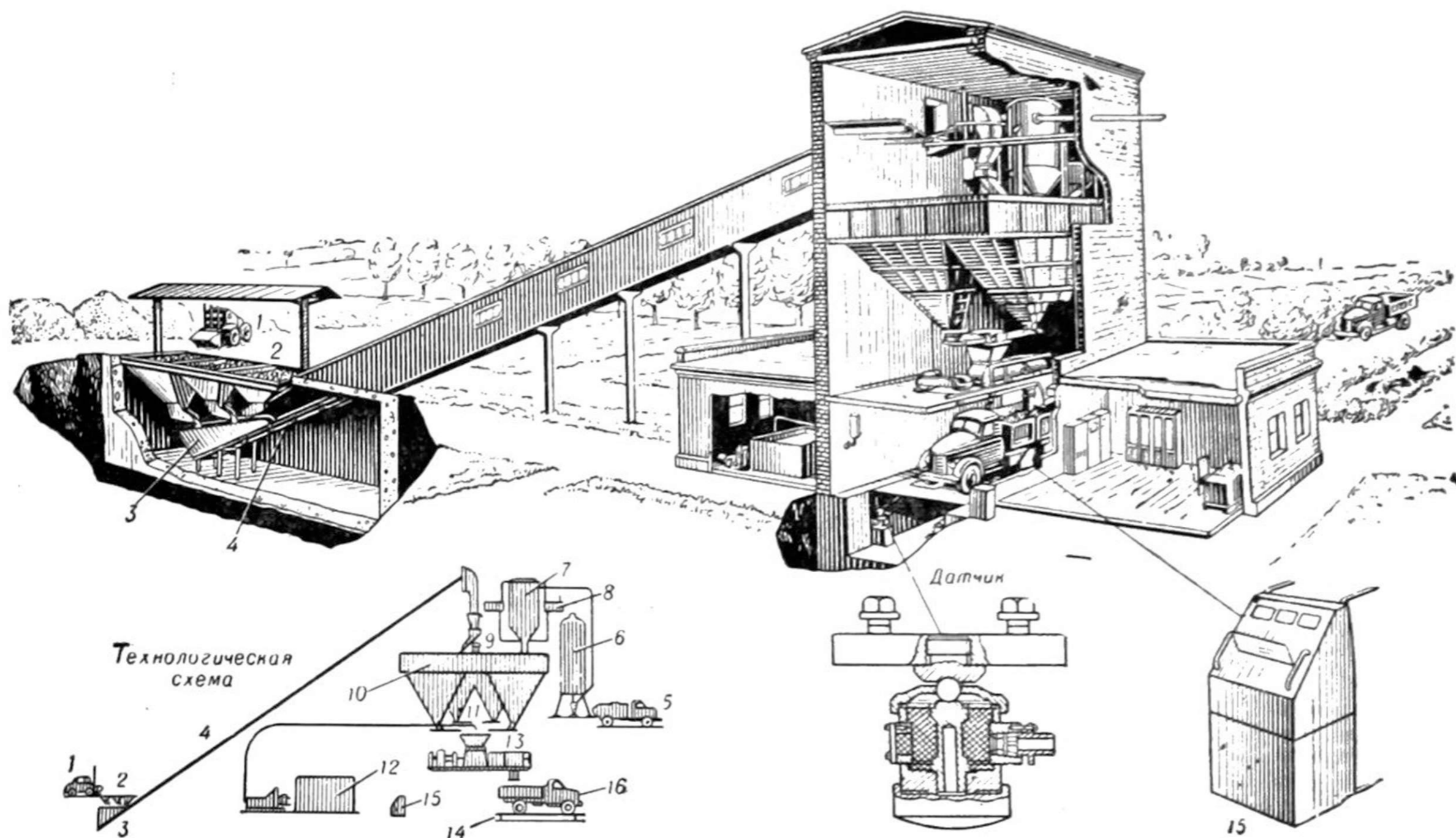
Схема бетонного завода-автомата: 1 — ковшовый погрузчик; 2 — приемный бункер; 3 — вибропитатель; 4 — ленточный транспортер; 5 — автоцементовоз; 6 — склад цемента; 7 — циклон; 8 — фильтровальное устройство; 9 — поворотная головка; 10 — расходные бункеры; 11 — дозаторы; 12 — дозатор для воды; 13 — смеситель; 14 — весовая платформа; 15 — программно-счетное устройство; 16 — автобетоновоз.
