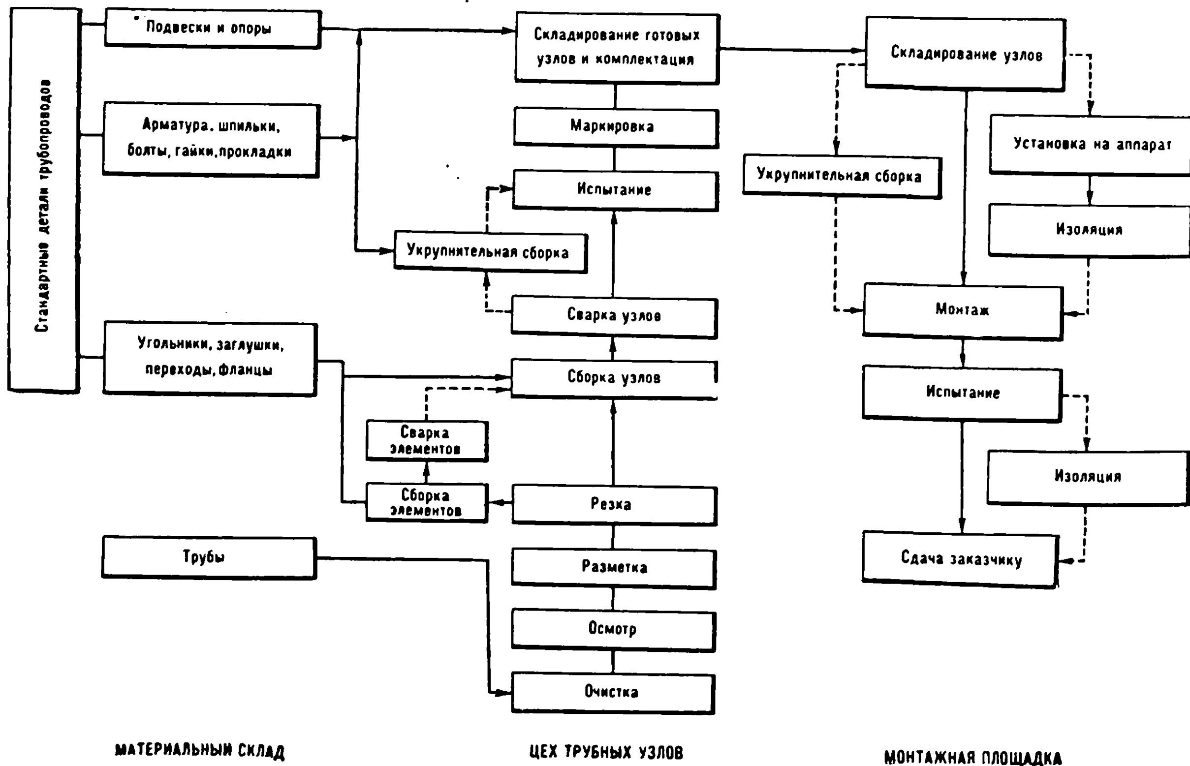
СХЕМА ИЗГОТОВЛЕНИЯ И МОНТАЖА УЗЛОВ ТРУБОПРОВОДОВ
