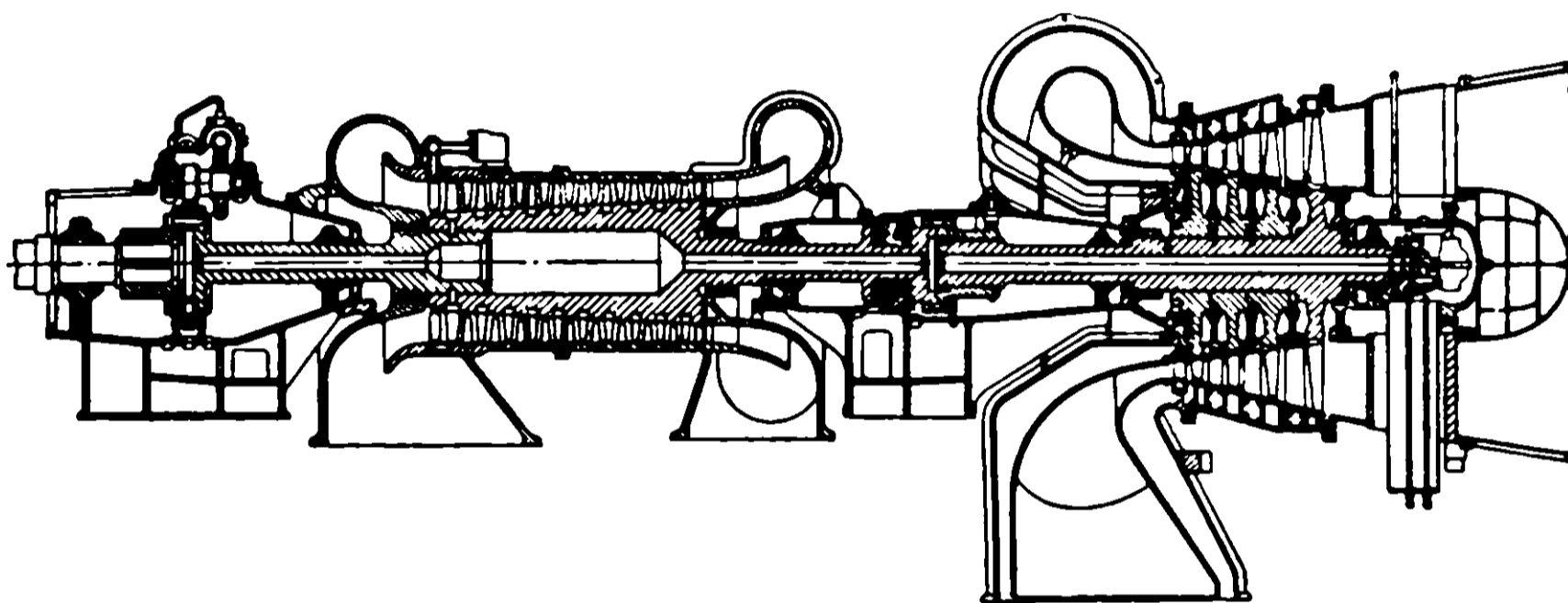
Рис. 2. Продольный разрез компрессора среднего давления и турбины низкого давления.
