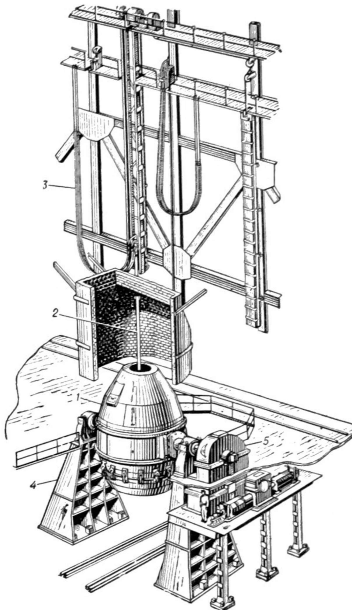
Рис. 1. Схема конвертера и подачи кислорода: 1 — конвертер; 2 — водоохлаждаемая фурма, по которой подается кислород; 3 — шланги для подачи воды и кислорода к фурме; 4 — станина конвертера; 5 — механизм наклона конвертера.
