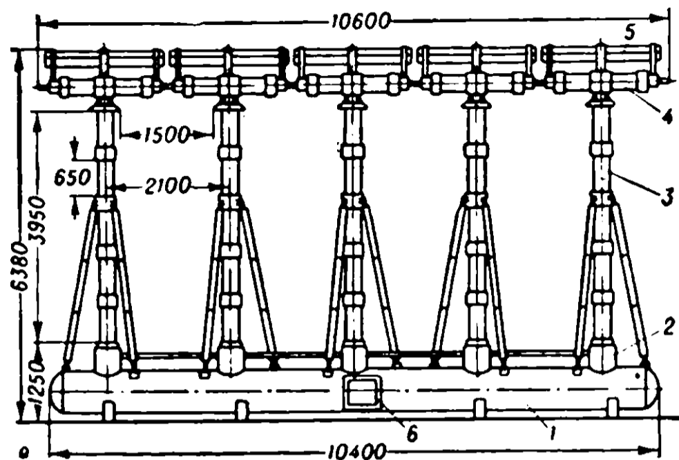
Фаза воздушнонаполненного выключателя 500 кВ, 2000 А, 25 000 Мва: а) расположение разрывов: 1 — резервуар, 2 — дутьевой клапан, 3 — опорные воздухопроводы, 4 — дугогасящие разрывы, 5 — емкостной делитель напряжения, 6 — шкаф управления, б) колонка с разрывами.
