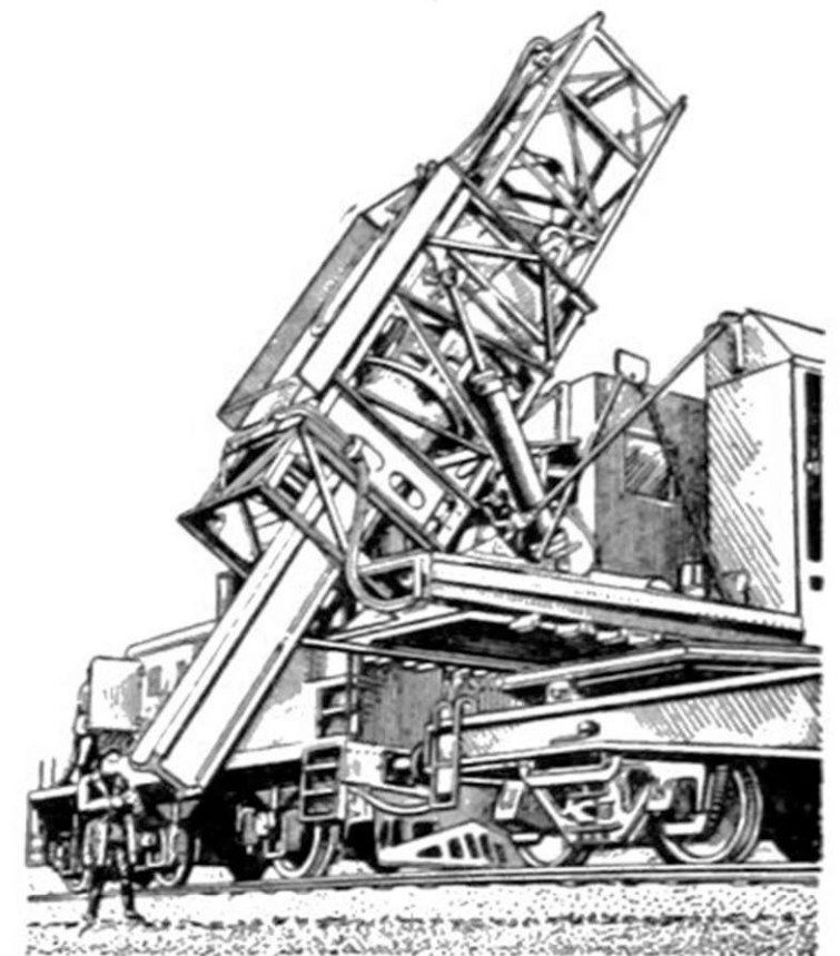
Рис. 3. Виброагрегат АВСЭ для погружения фундаментов опор.
