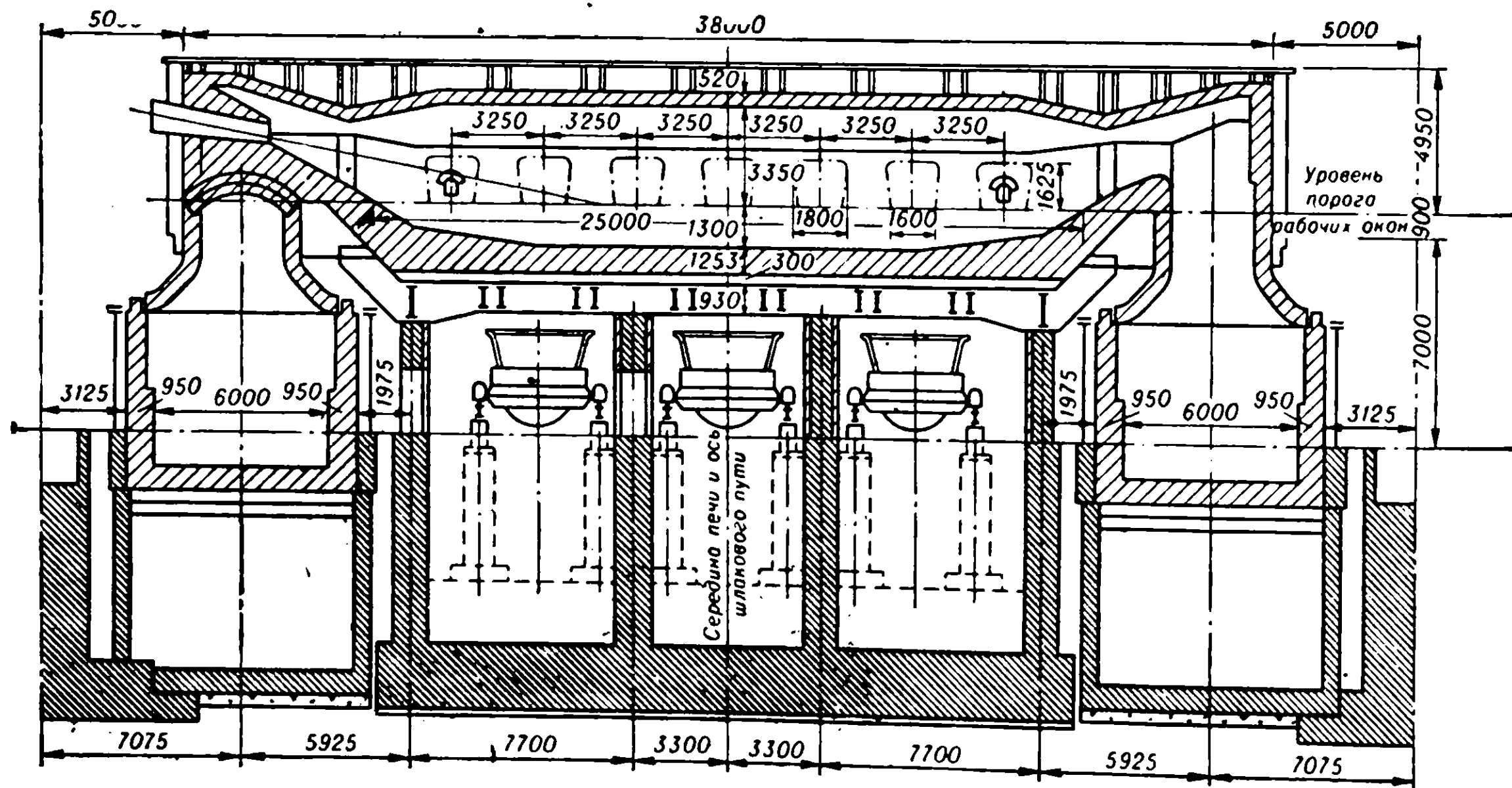
Схема 900-тонной мартеновской печи.
