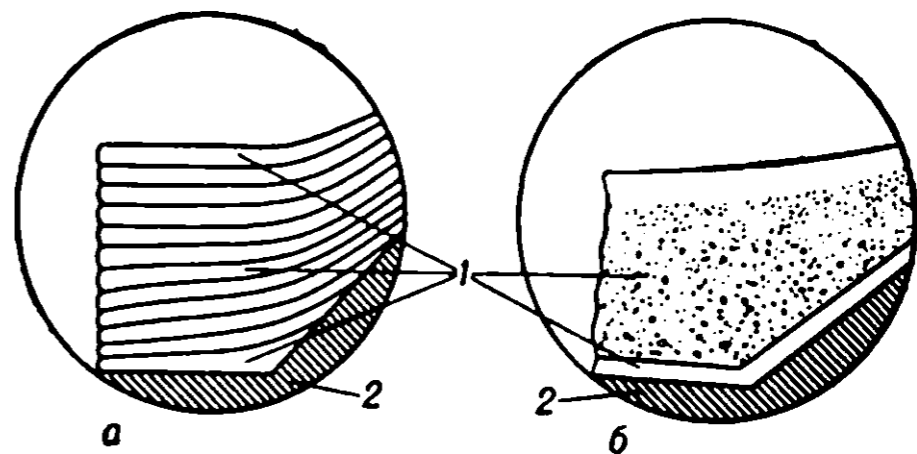
Рис. 2. Схема наварки новой подины (перед первой плавкой): а — по старому способу; б — по новому способу; 1 — слой наварки; 2 — магнезитовая кладка.
