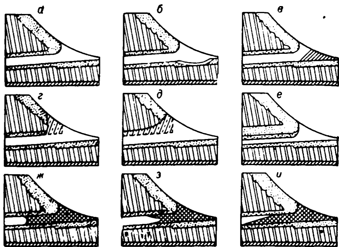
Рис. 1. Схемы сталевыпускного отверстия в разных состояниях: а — нормальные; б — яма в устье отверстия; в — порог перед отверстием; з — оборвана верхняя часть отверстия; д — короткое и широкое отверстие; е — узкое и длинное отверстие; ж — отверстие при правильной разделке; з, и — отверстия при неправильной разделке.
