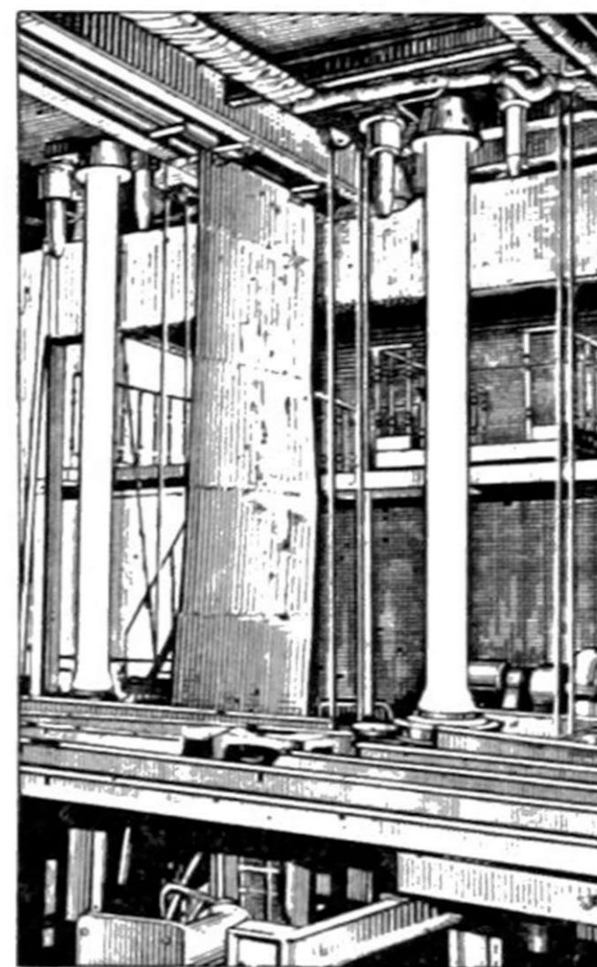
Рис. 2. Отливка водопроводных труб полу непрерывным способом. Вид первого этажа.
