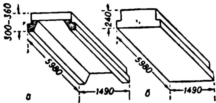
Рис. 1. Плиты из ячеистого бетона для покрытий промышленных зданий: а — ребристые («КАП»), б — плоские («ГКП»).
