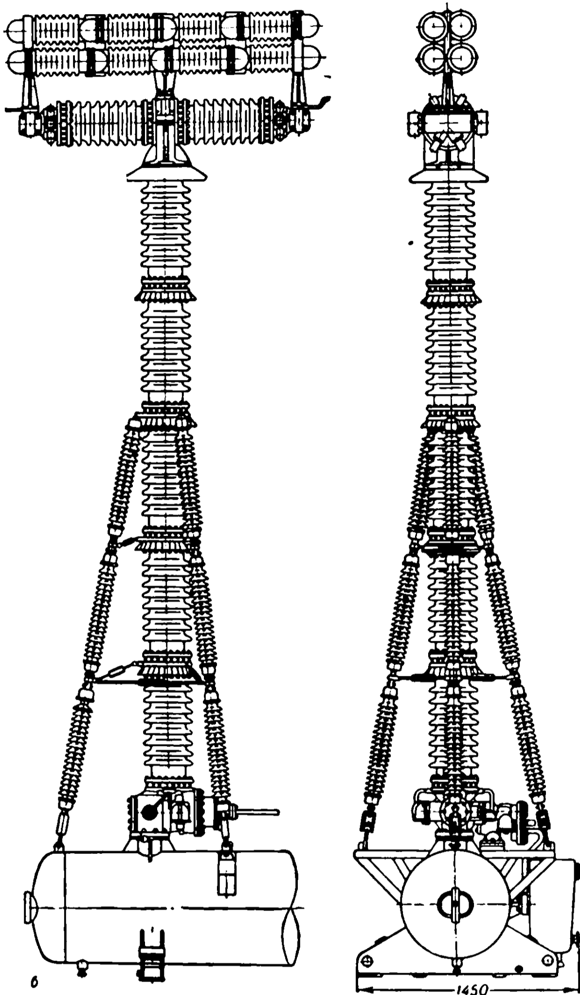
Фаза воздушнонаполненного выключателя 500 кВ, 2000 А, 25 000 Мва: а) расположение разрывов: 1 — резервуар, 2 — дутьевой клапан, 3 — опорные воздухопроводы, 4 — дугогасящие разрывы, 5 — емкостной делитель напряжения, 6 — шкаф управления, б) колонка с разрывами.
