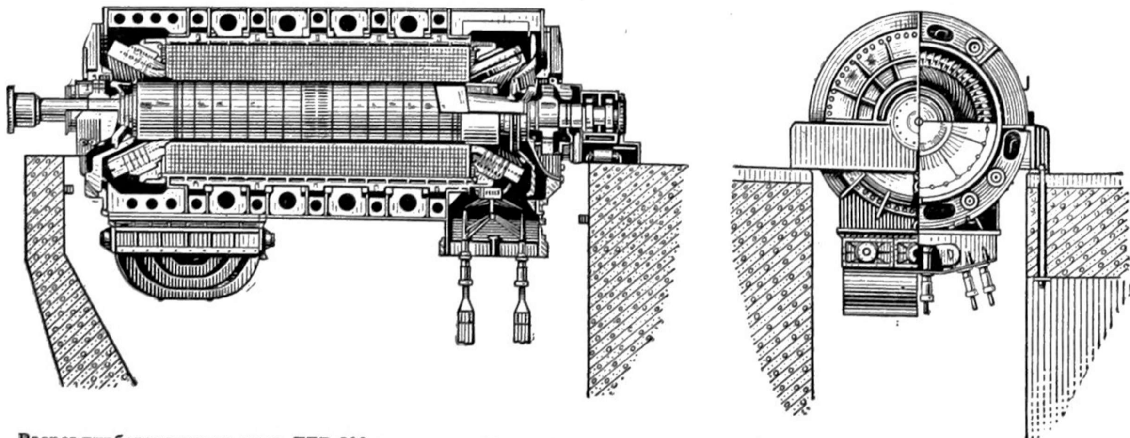
Разрез турбогенератора типа ТГВ-300 мощностью 300 тыс.квт Харьковского завода «Электротяжмаш» им. В. И. Ленина.
