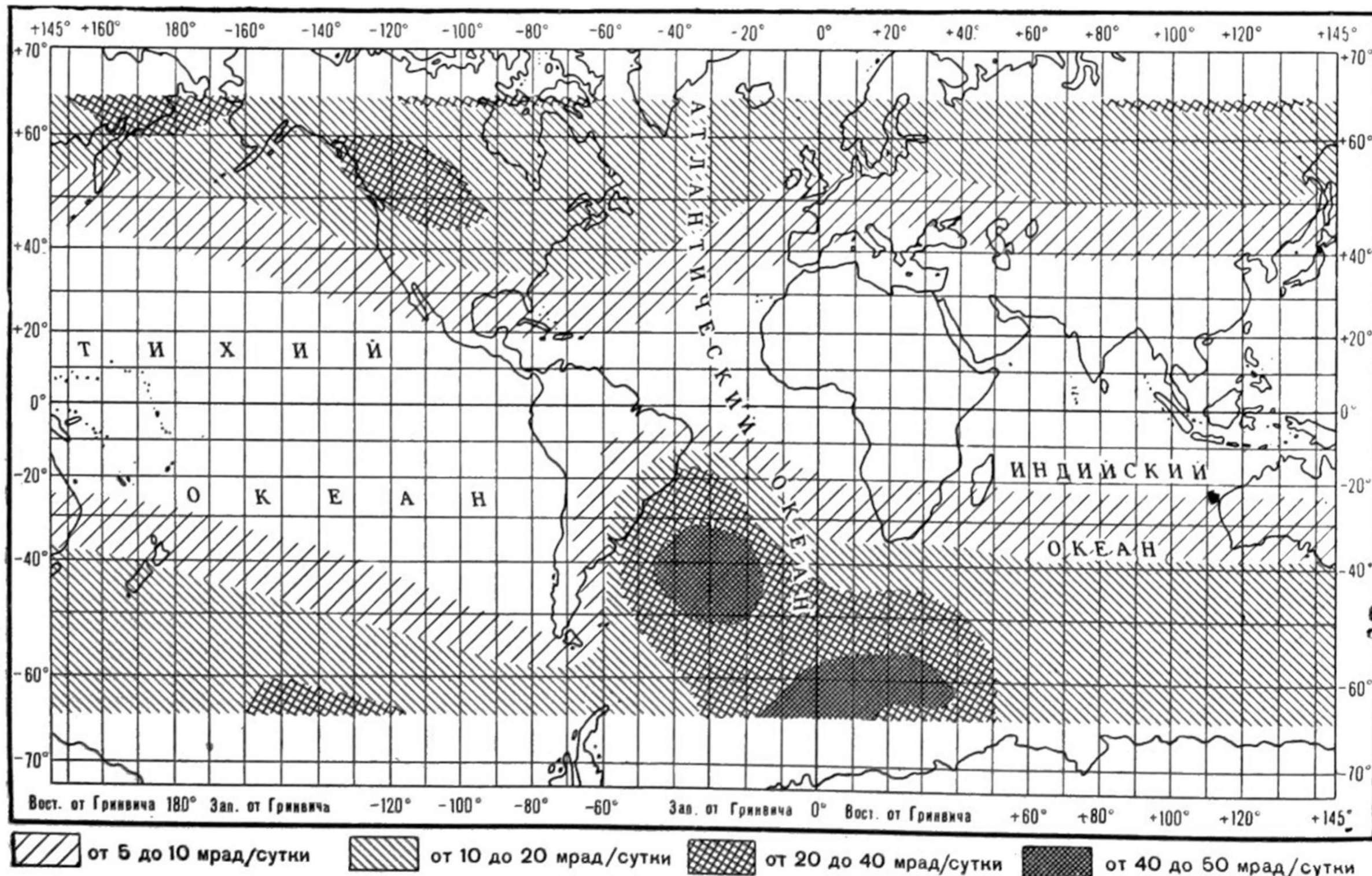
Схема зон повышенной интенсивности излучения на высоте ~320 км от Земли.
