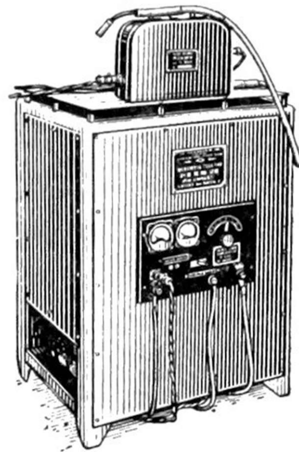
Полуавтомат А-547 для сварки в углекислом газе с выпрямителем ВС-300 (конструкция Ин-та электросварки им. Е. О. Патона).
